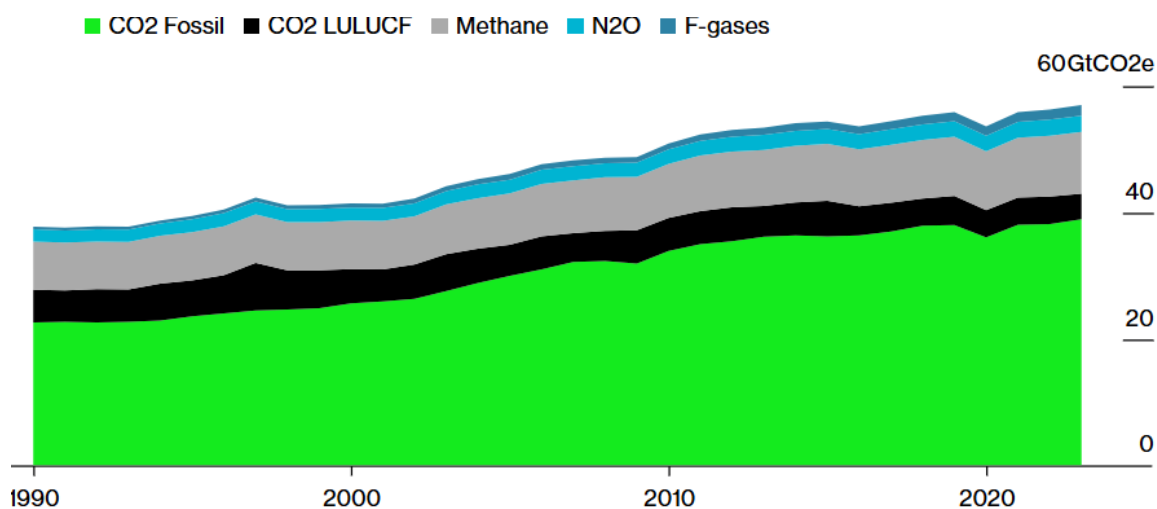
شکل ۱: نمودار انتشار دی‌اکسید کربن ناشی از مصرف سوخت‌های فسیلی از سال ۱۹۹۰ تا ۲۰۲۴
